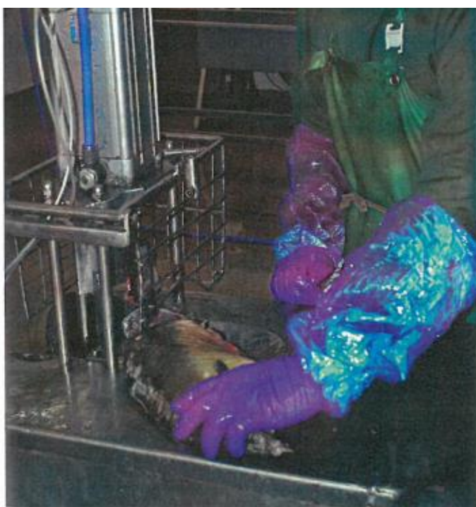
Obr. č. 5: Oddělení hlavy ryb pomocí gilotinového nože (foto František Ježek)
